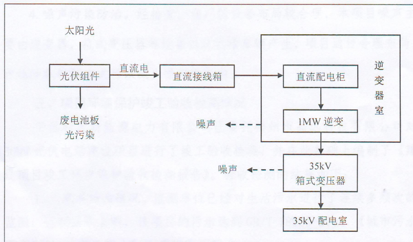
生产工艺及产污环节图
